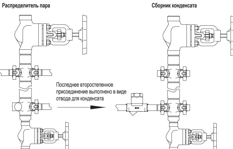
... с основным запорным клапаном и второстепенными присоединениями аналогично сборнику конденсата - исполнение со сливным клапаном
