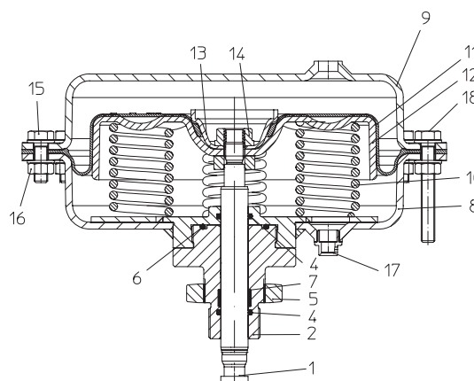
Пневмопривод ARI-FA Пружина открывает
