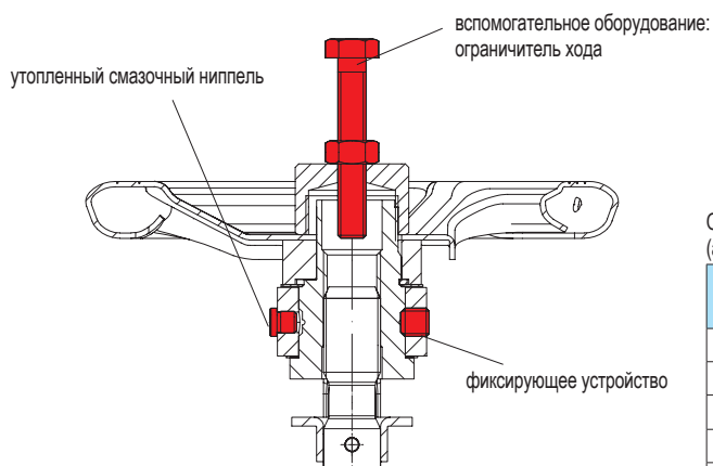
Утолщенный смазочный ниппель / фиксирующее устройство / ограничитель хода (только Конструкция FABА-Plus и FABА-Supra с цельным штоком)
