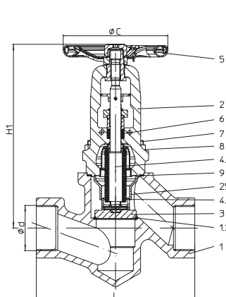
Фиг. 149....111....2 с резьбовыми муфтами цельный шток
